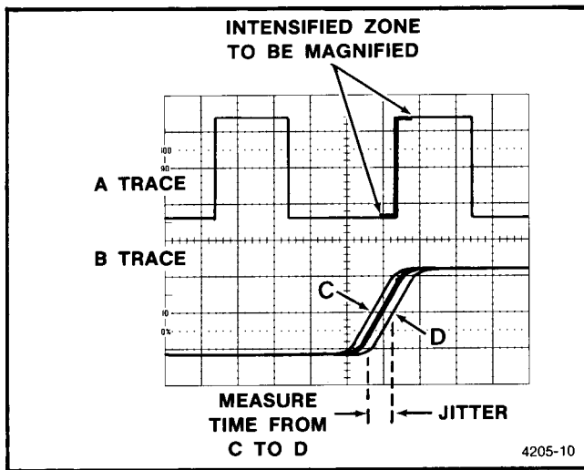
Fig. 4-6. Pulse jitter.
